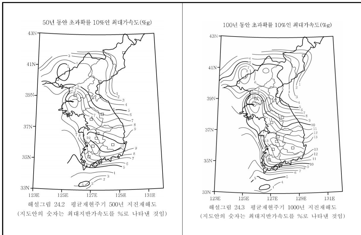
【그림 6.12】 평균재현주기 500년 및 1000년 지진재해도
