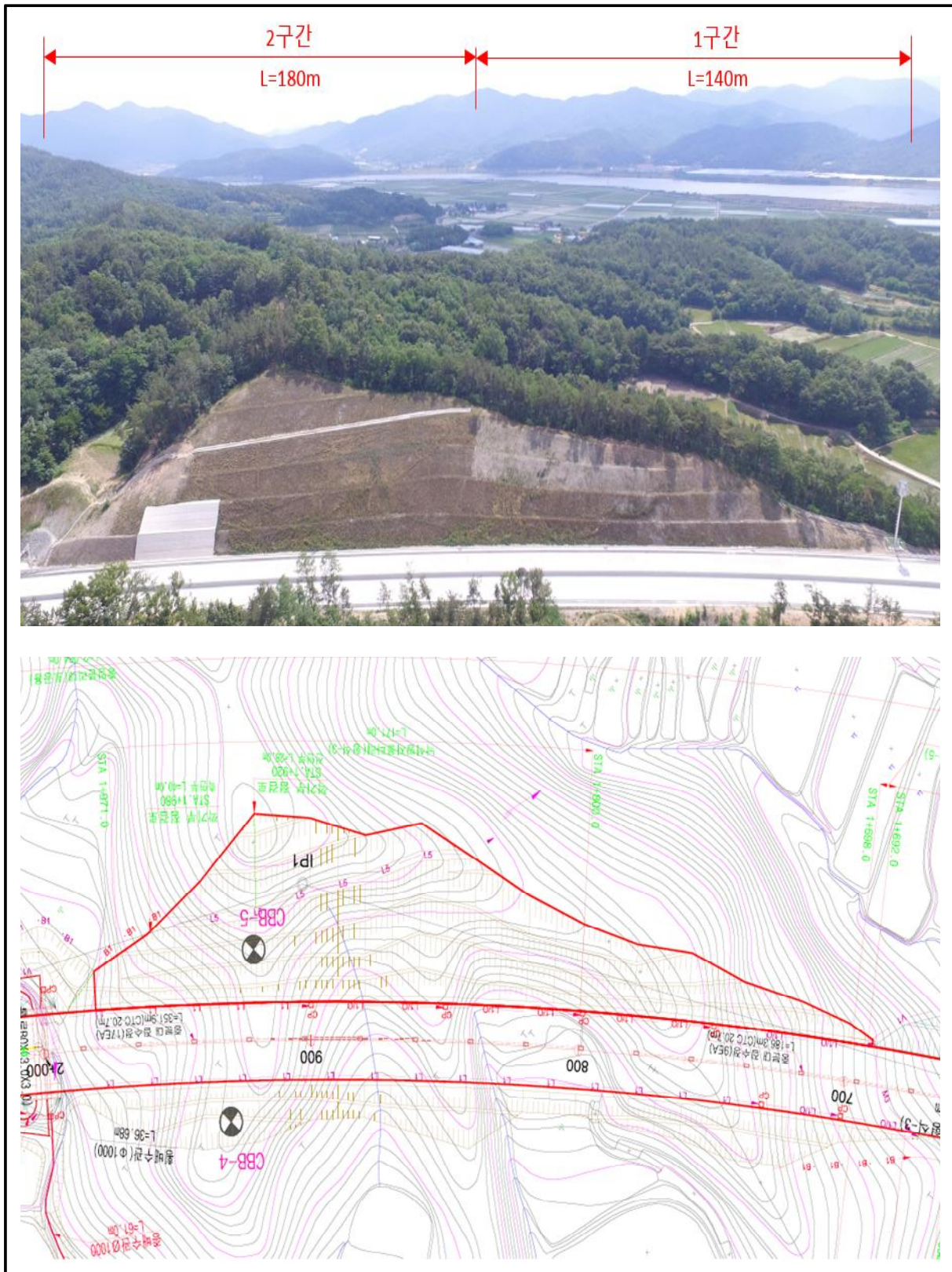
【그림 6.14】 영천절토06 검토대상 비탈면구간
